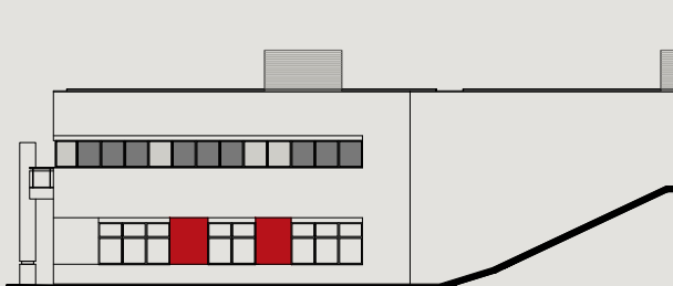
FAÇADE EST
